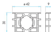
Адаптер Adapter
