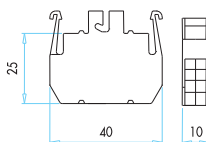
Блок-контакт подсветки серии В с неоновой лампой Neon Lamp Mountable B Series Light Block
