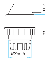
Переключатель Selector
